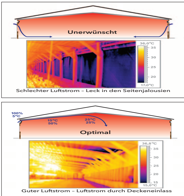
Abbildung 13. Luftstrom
